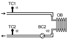
Рисунок 4.1 Модифицированная схема потребления СП10
