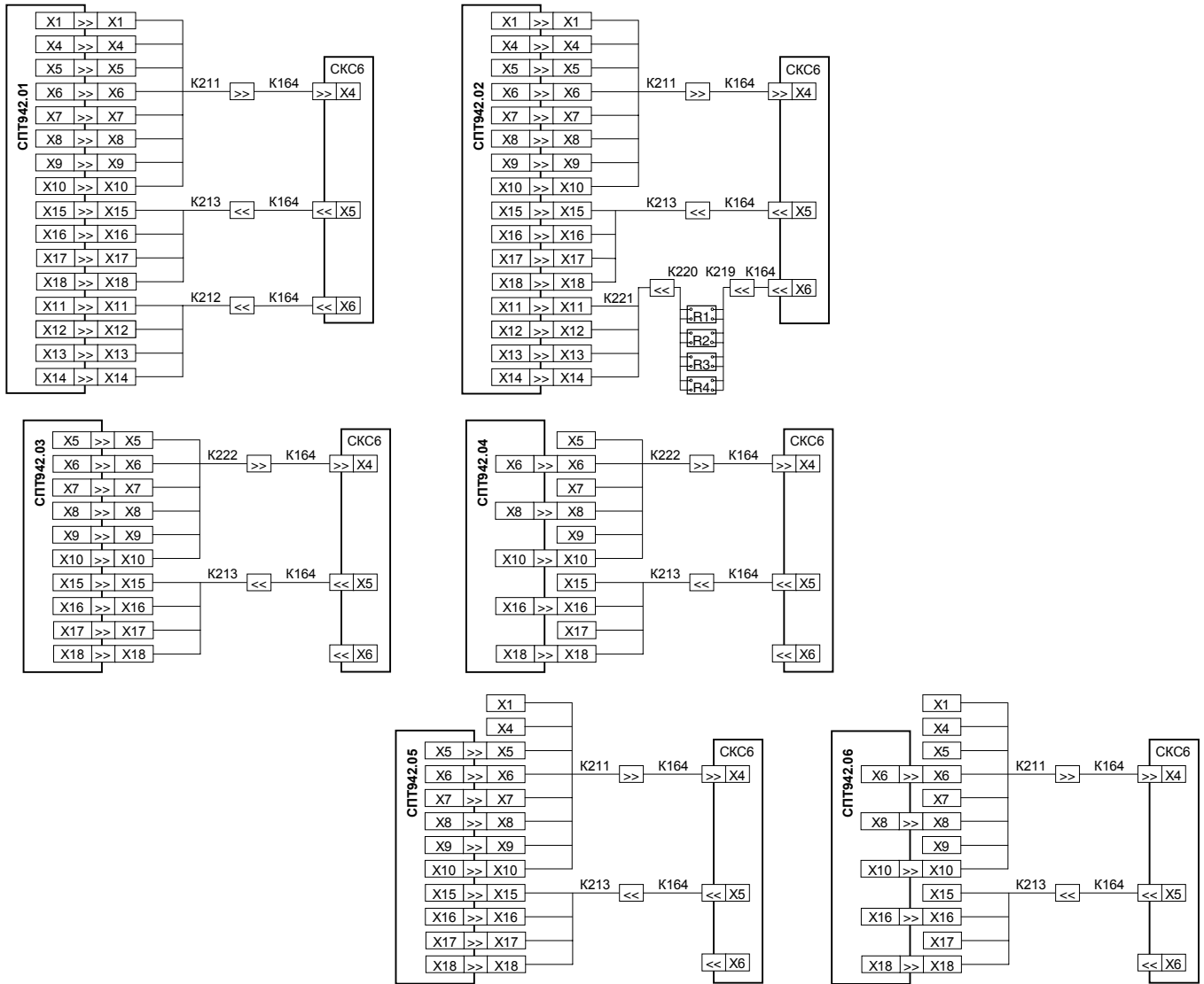
Рисунок 10.1 Схемы поверки
