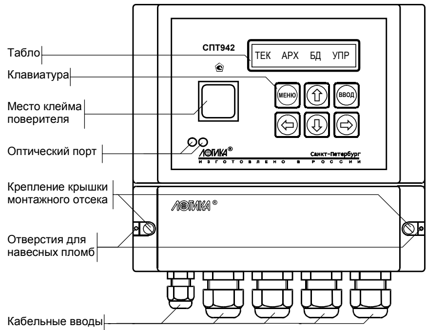
Рисунок 3.1 Вид спереди
