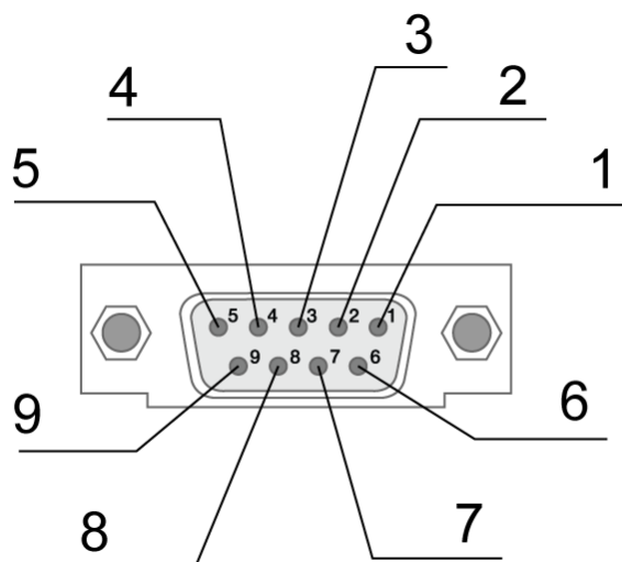
Рис. 2.3. Интерфейсный разъем
