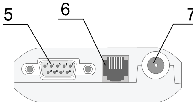
Рис. 2.2. Вид сзади
